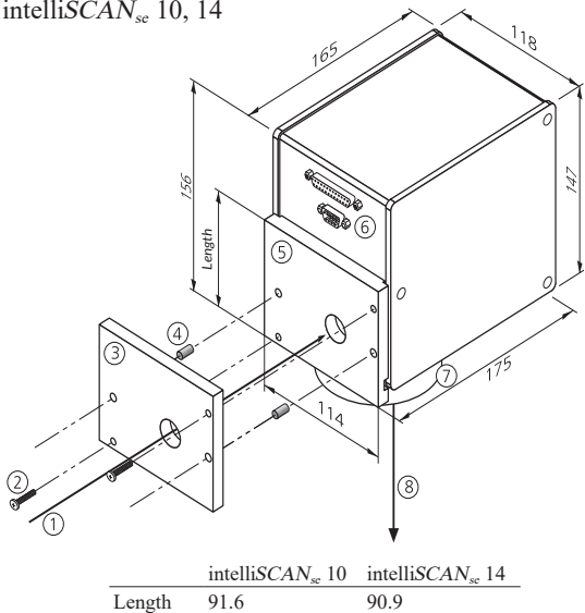
intelliSCAN sc 10, 14
